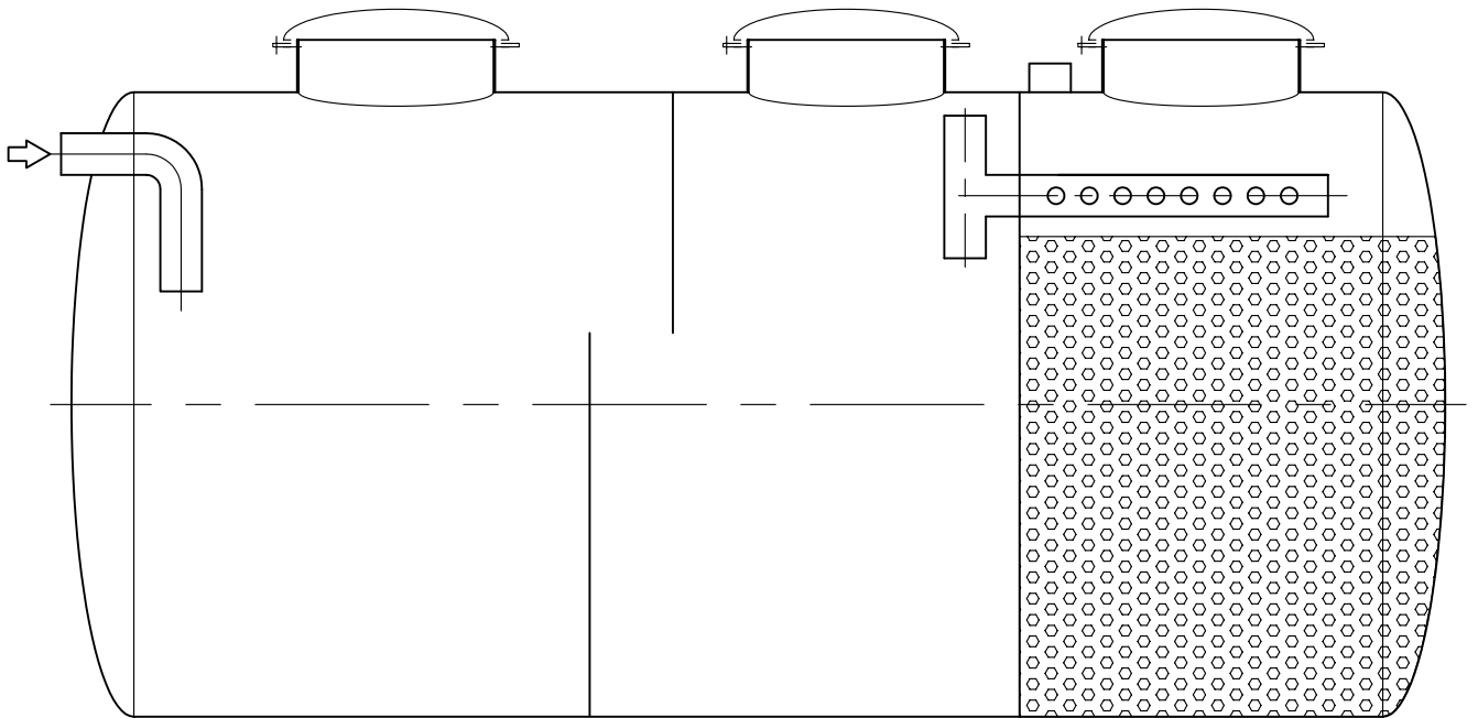
Sección
